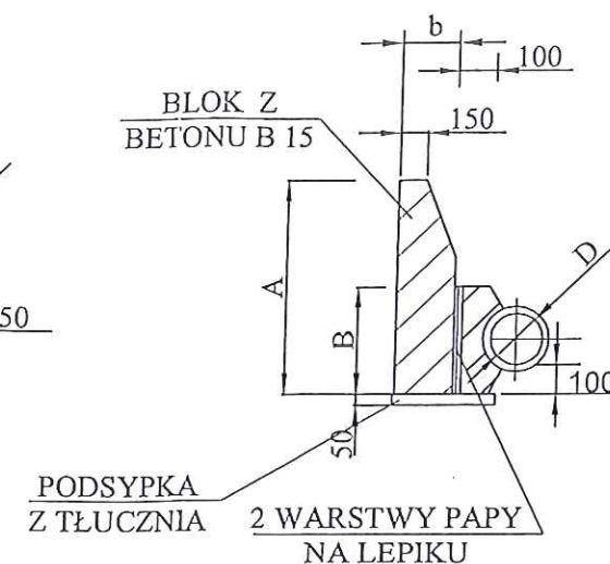
BLOK OPOROWY BETONOWY PRZY \varnothing 200 - 300
