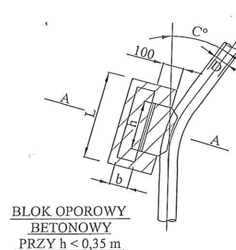
WYMIARY BLOKÓW OPOROWYCH
