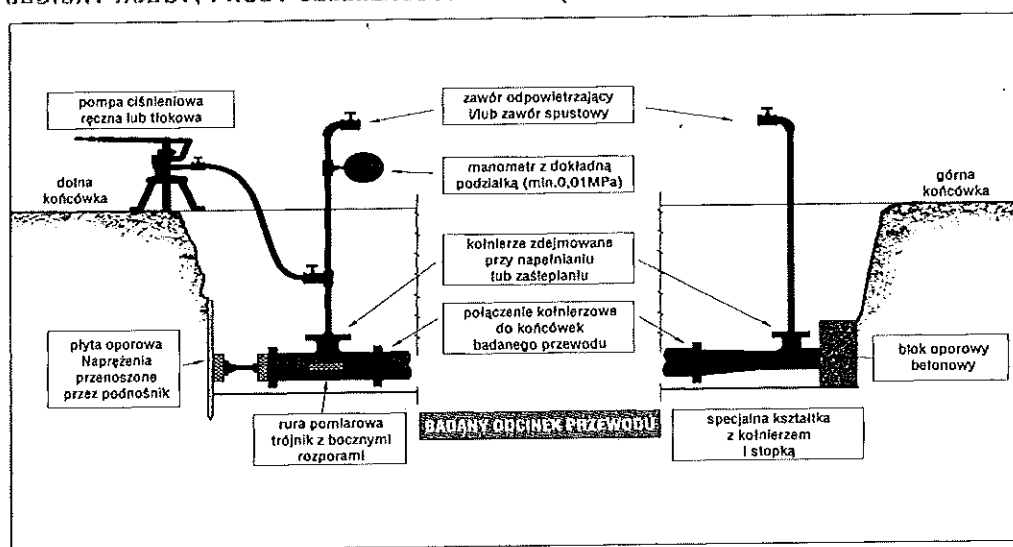
Schemat instalacji do próby szczelności
