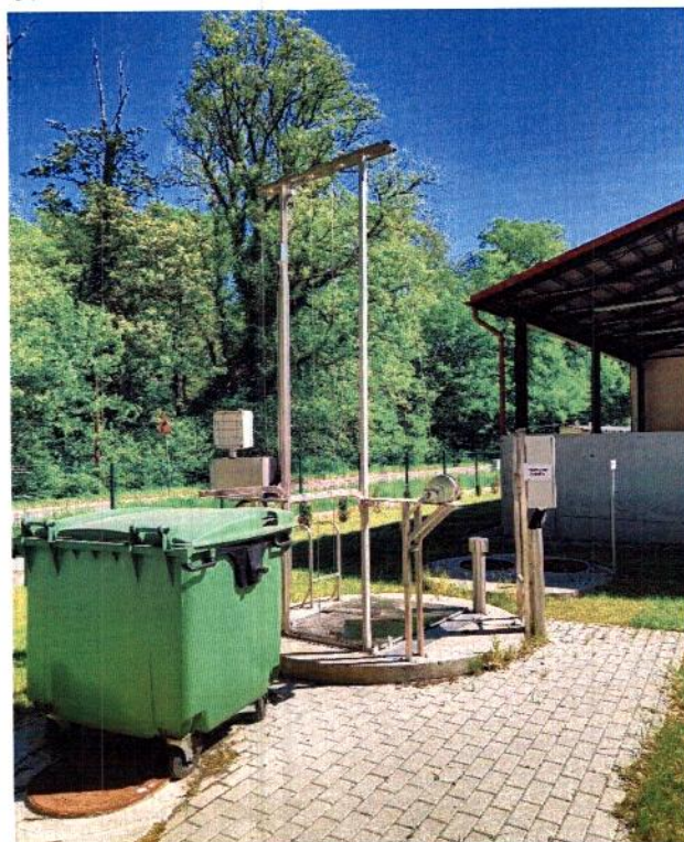
Zdjęcie nr 2. Pompownia ścieków
