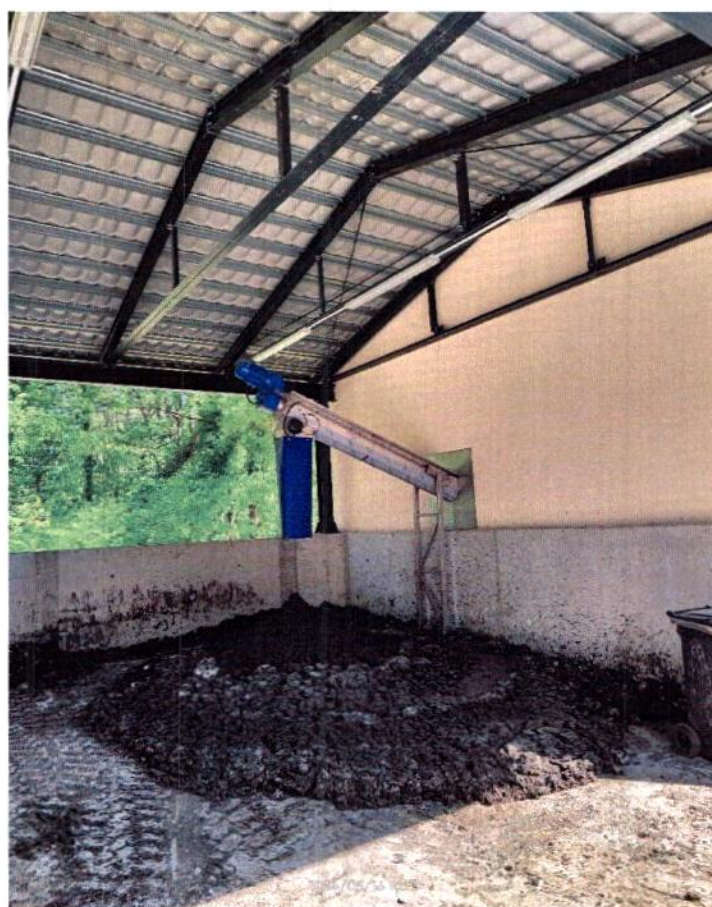
Zdjęcie nr 6. Wiata na odwoniony osad
