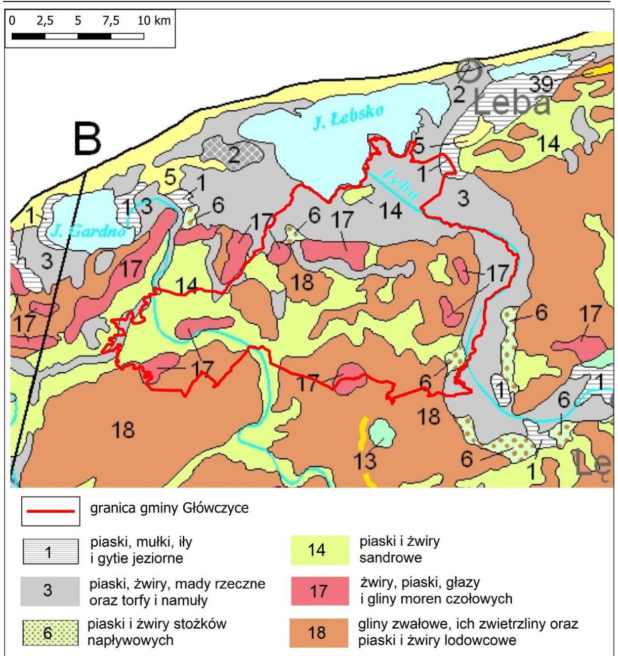
Rys. 6. Obszar gminy Główczyce na tle Mapy geologicznej Polski 1:500 000.
