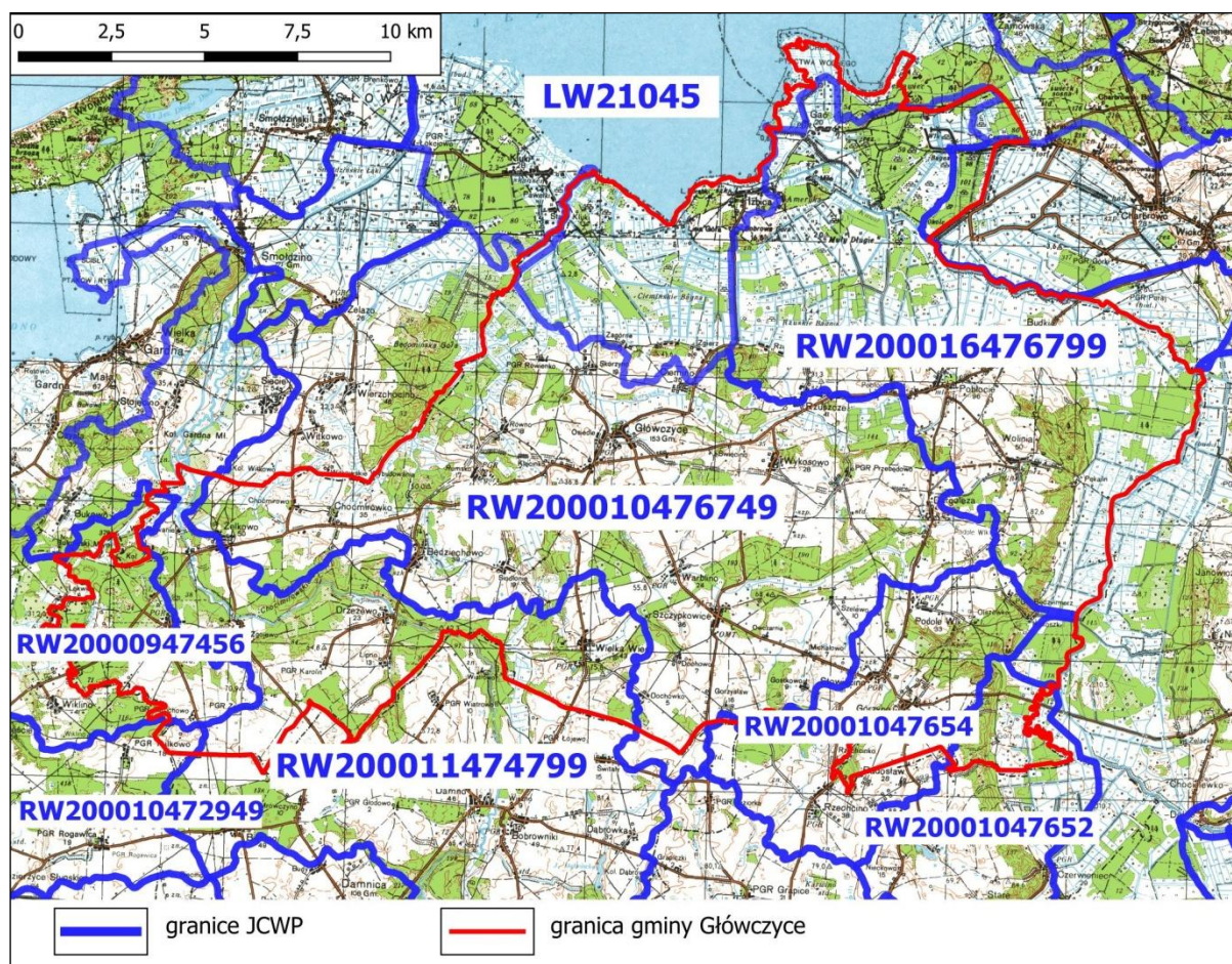
Rys. 9. Położenie gminy Głowczyce na tle podziału na tle podziału na jednolite części wód powierzchniowych. Źródło: dane apgw.gov.pl
