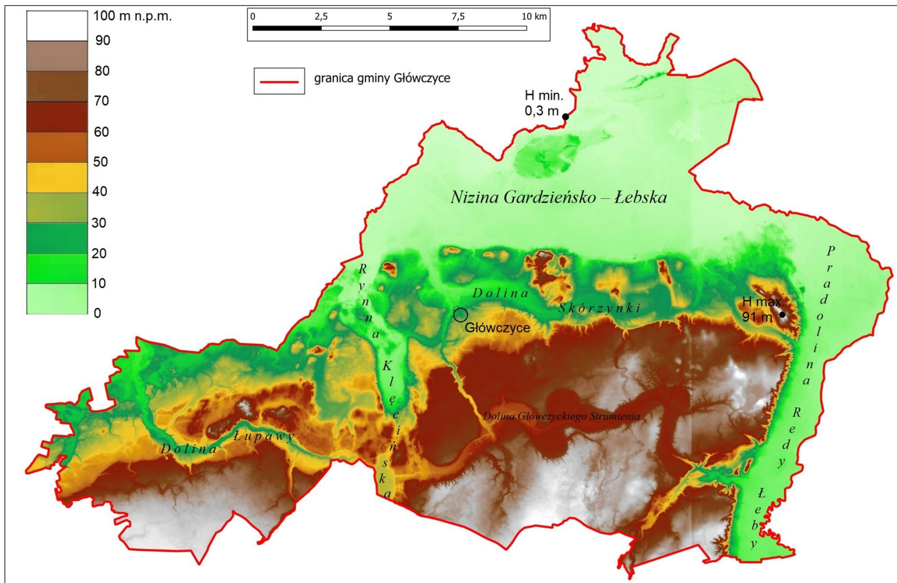
Rys. 8. Ukształtowanie powierzchni terenu obszaru gminy Główczyce. Źródło: opracowanie własne, dane geoportal.gov.pl
