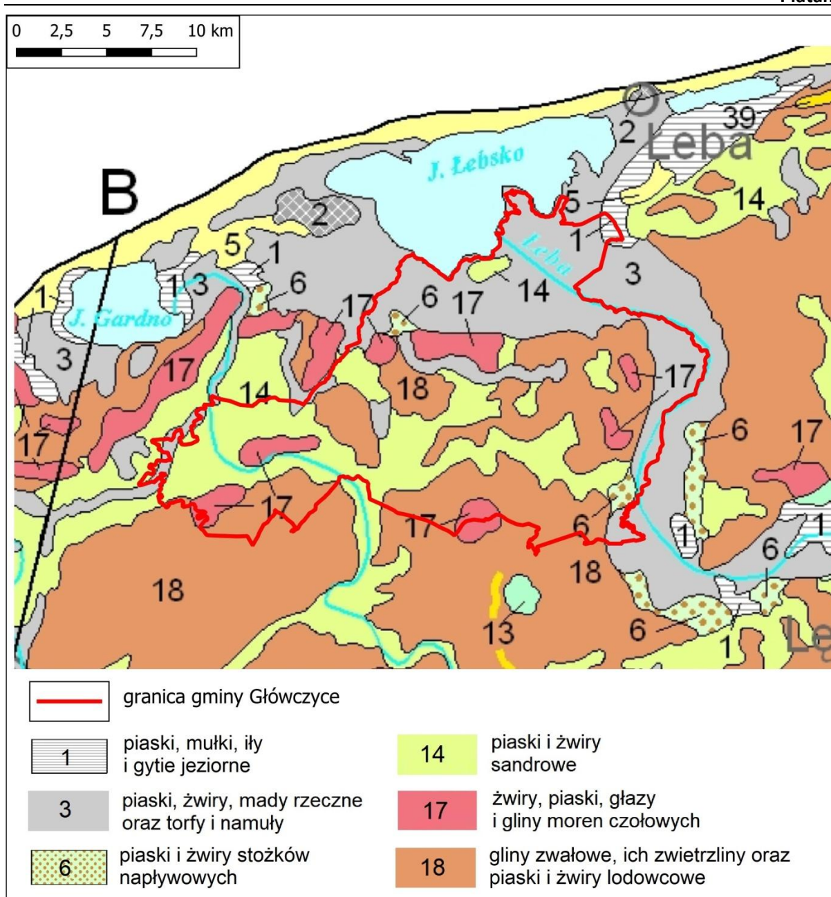
Rys. 6. Obszar gminy Głowczyce na tle Mapy geologicznej Polski 1:500 000.
